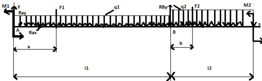
Рис. 6. Расчетная схема балки.
