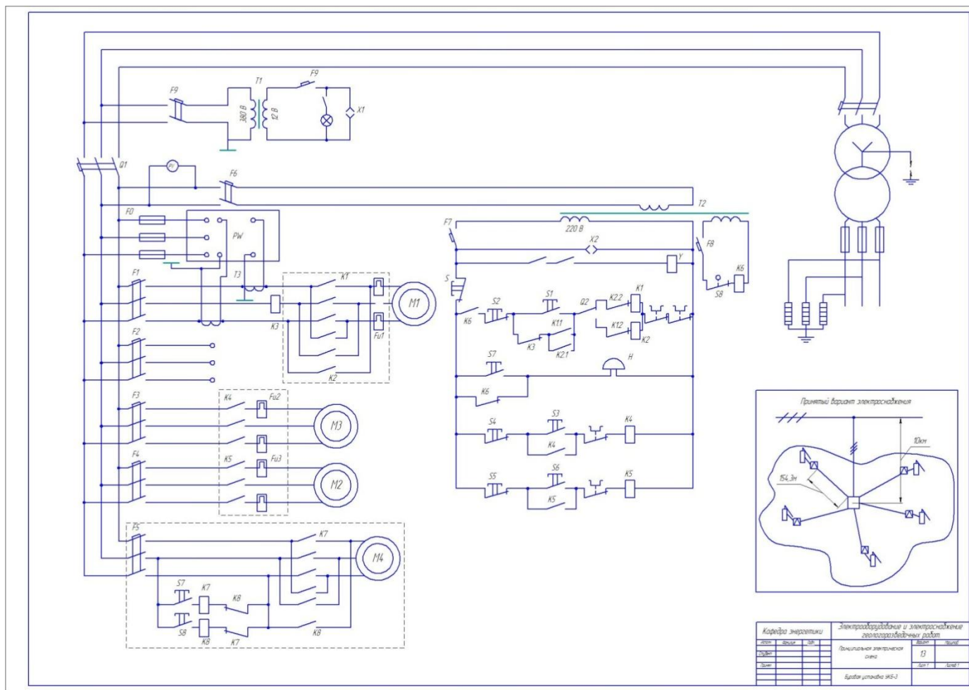
Рисунок 10.15 – Схема электрическая
